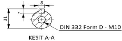
KESİT A-A
